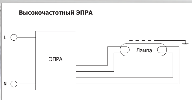
Одиночное подключение
